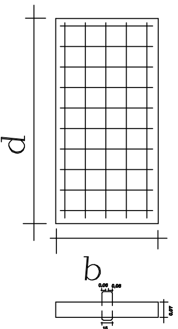
DETALHE DA TAMPA
