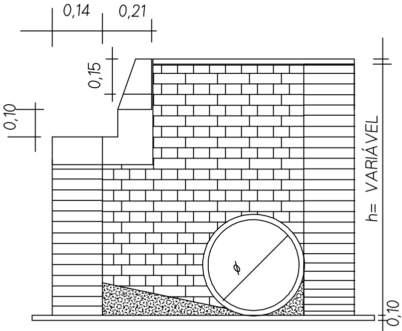
SEÇÃO AA
