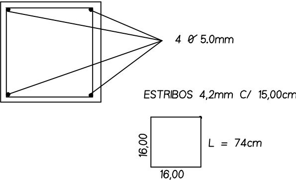
CINTA DE COROAMENTO
