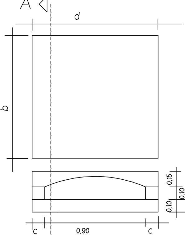
PLANTA BAIXA
