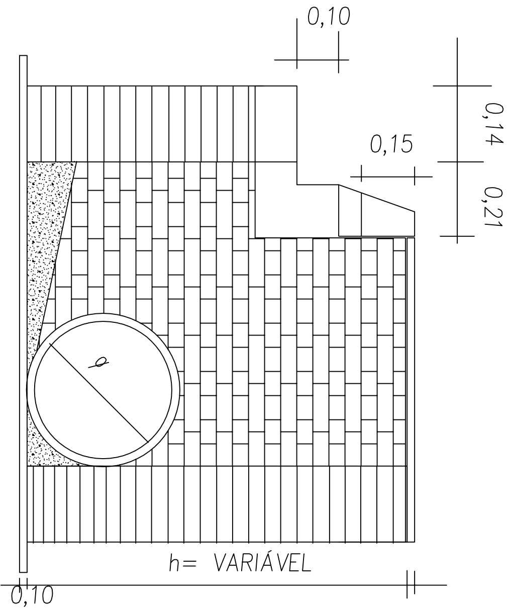
SEÇÃO AA
