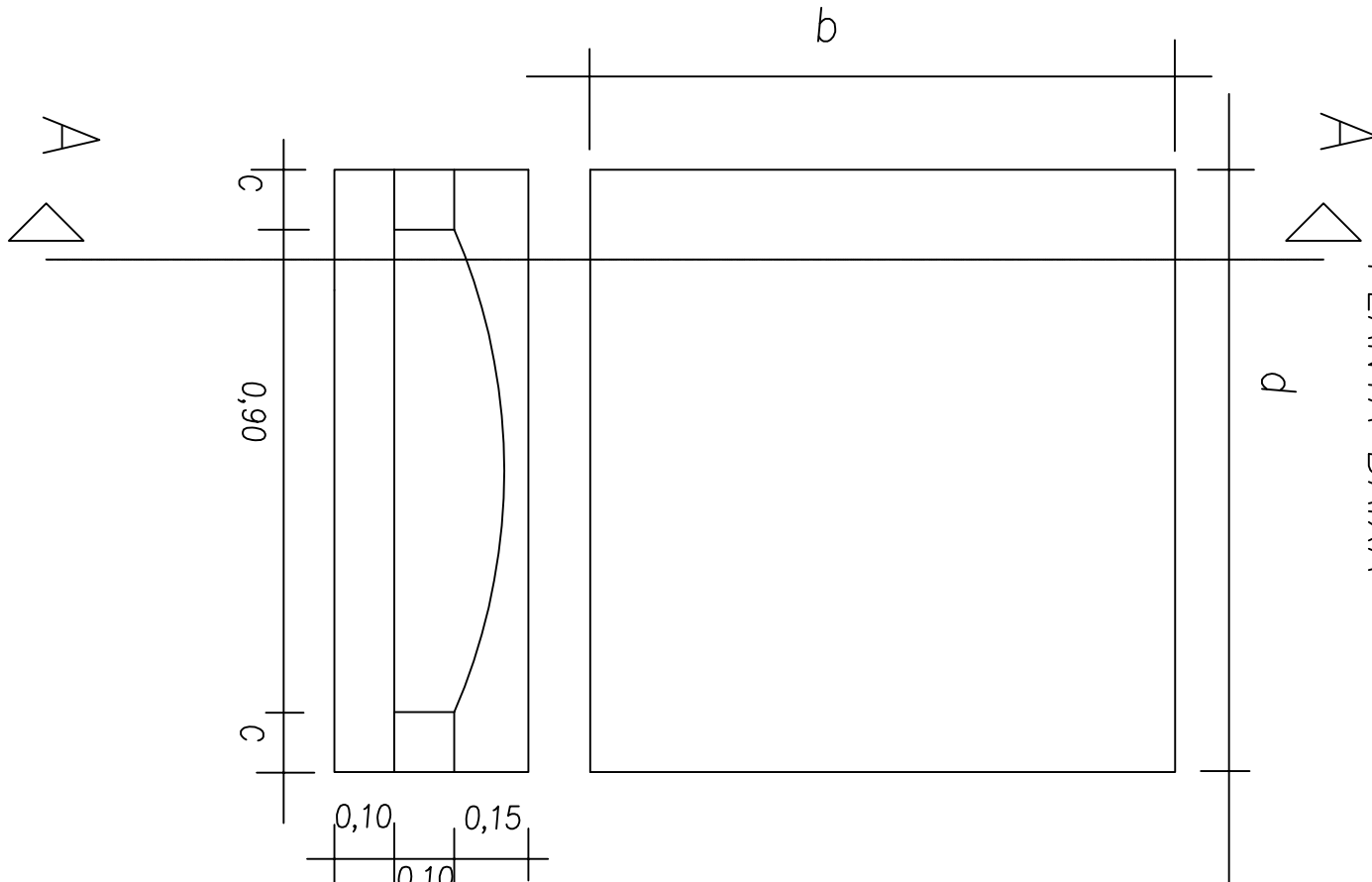
PLANTA BAIXA
