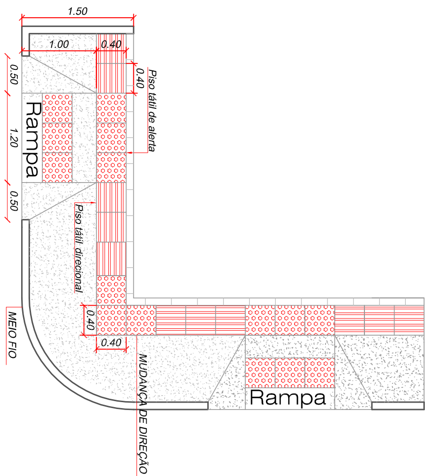
Detalhe Passeio Esc. 1:50
